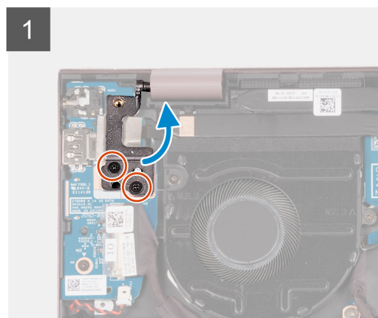
2x M2.5x4
